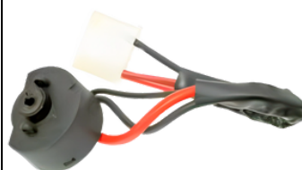
Interruptor de Ignición Con 3 Salidas Chevette MZ23064
